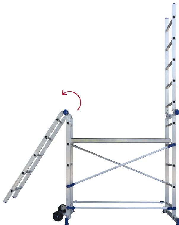
Sistema exclusivo de articulación hacia el exterior que permite no desmontar la parte baja del andamio Sistema exclusivo de articulação para o exterior que permite que a parte inferior do andaime não seja desmontada
