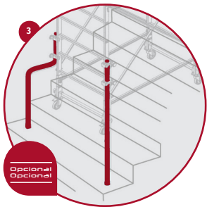
3 Estabilizadores fijados con abrazaderas de aluminio Estabilizadores fixados com grampas de alumínio
